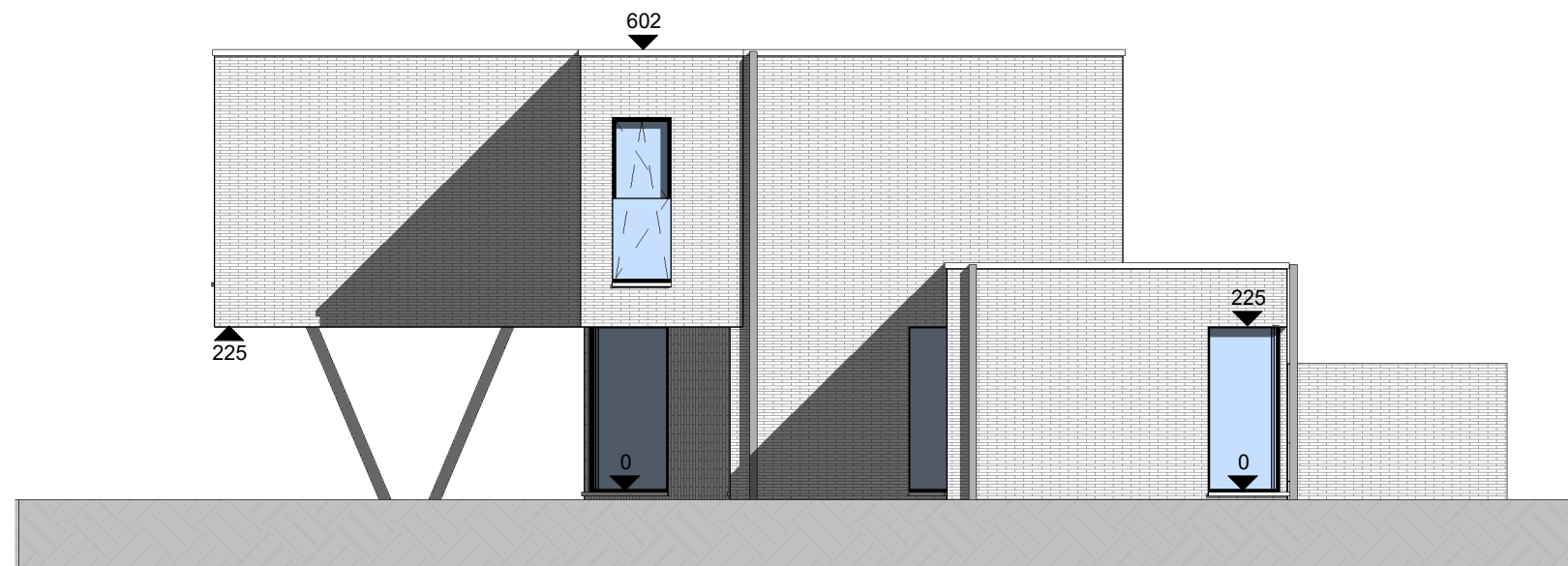
③ Rechter zijgevel woning 9 1 : 100
